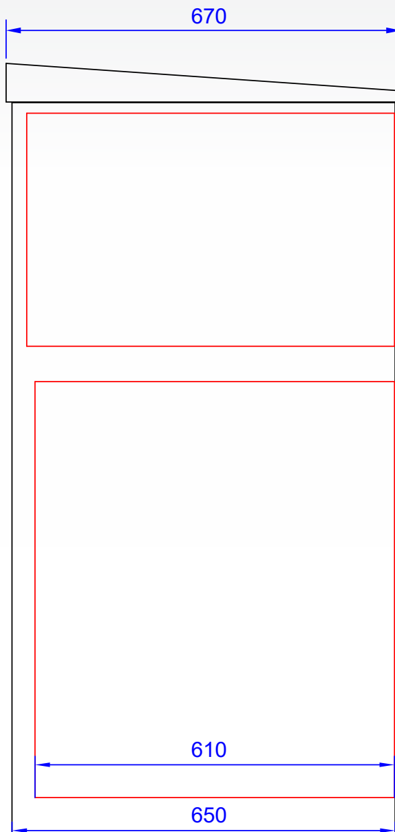
Seitenansicht
