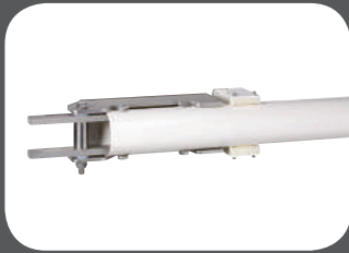
■ Balkenfixierung für Balken oval, ausschwingend
